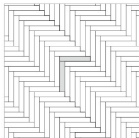
■C 铺贴引导图
